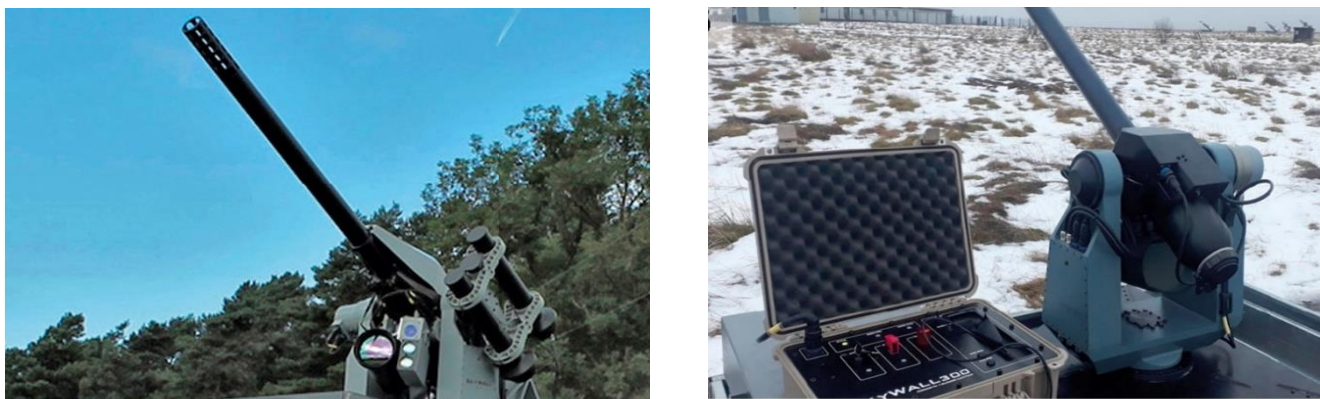
Рис.3 – Пневматическая турель для запуска снаряда с противодроновой сетью-ловушкой
